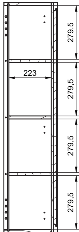
B-B ( 1:10 )
