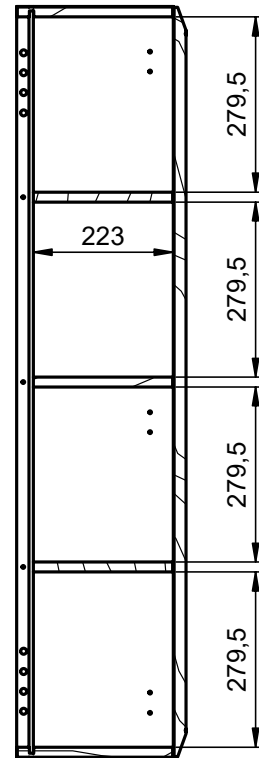
B-B ( 1:10 )
