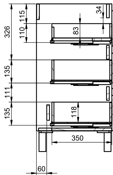
B-B ( 1 : 10 )
