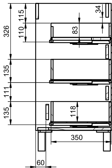
B-B ( 1 : 10 )
