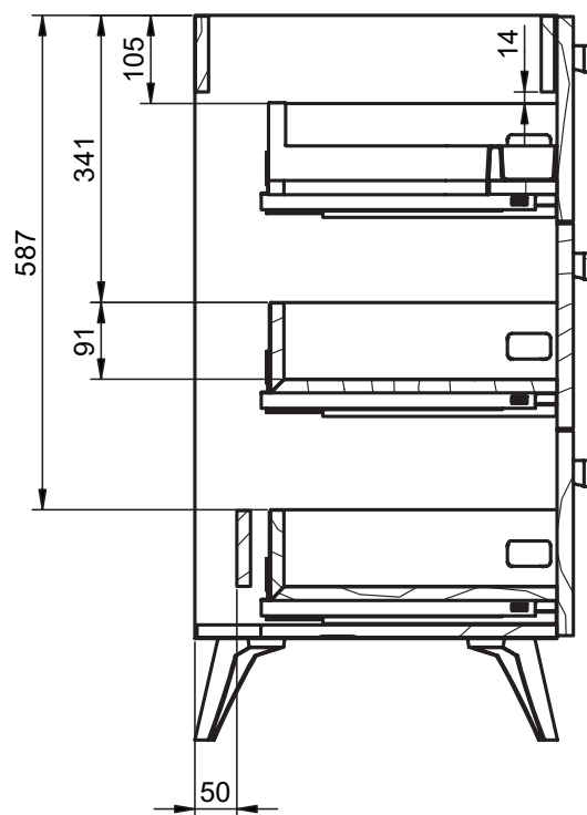
B-B ( 1 : 8 )
