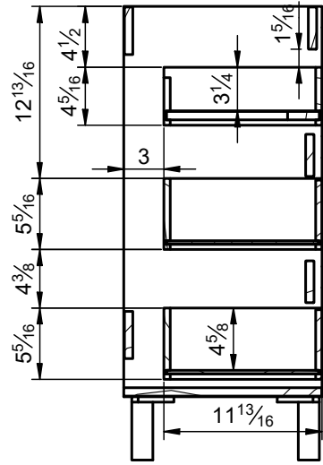
B-B ( 1 : 10 )
