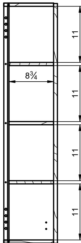
B-B ( 1:10 )
