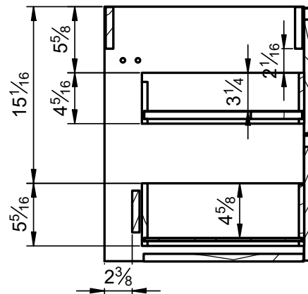
B-B ( 1 : 10 )
